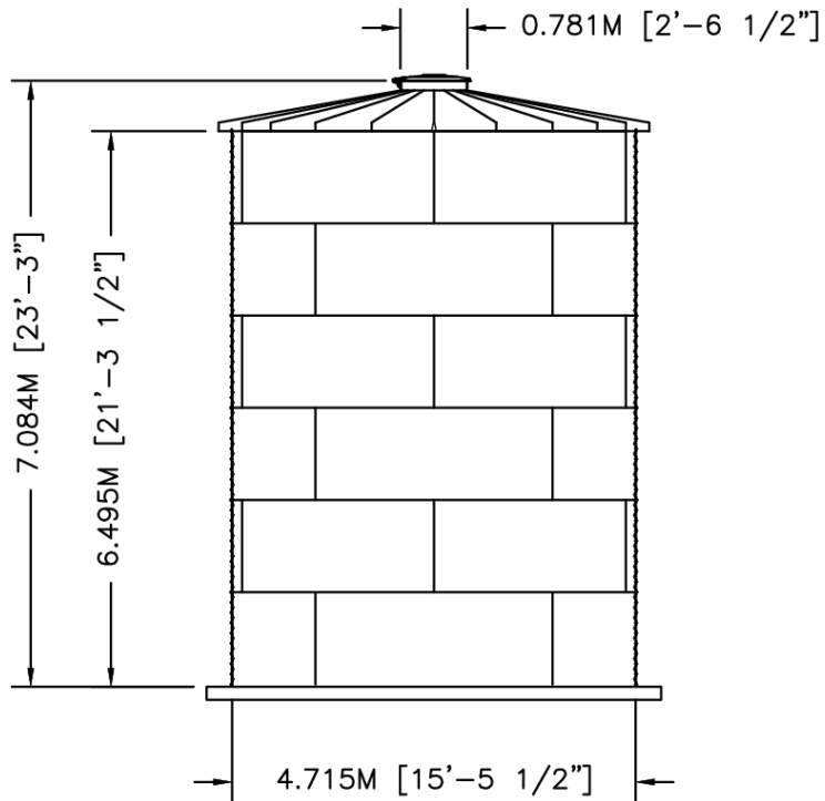
ELEVATION
